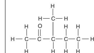
or \text{CH}_3\text{COCH}(\text{CH}_3)\text{CH}_2\text{CH}_3 3-methylpentan-2-one
