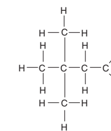
\text{CH}_3\text{C}(\text{CH}_3)_2\text{CH}_2\text{CHO} 3,3-dimethylbutanal
