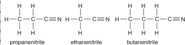
propanenitrile ethanenitrile butanenitrile
